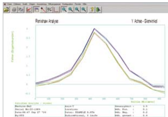
Стандартный вид результатов угловых измерений, представленных в виде графика.
