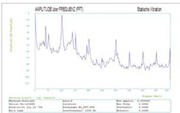
Частотный анализ по методу быстрого преобразования Фурье
