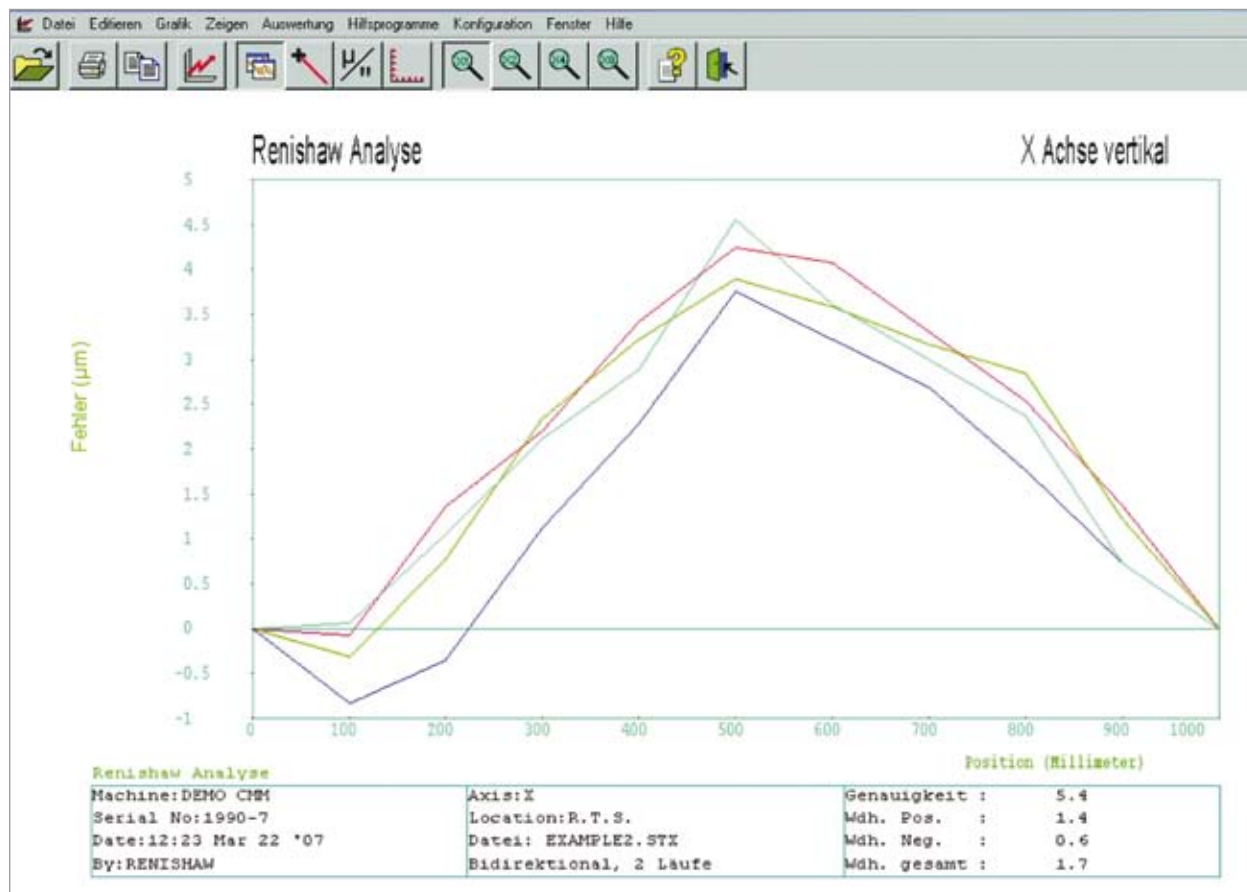
Стандартный вид результатов проверки прямолинейности
